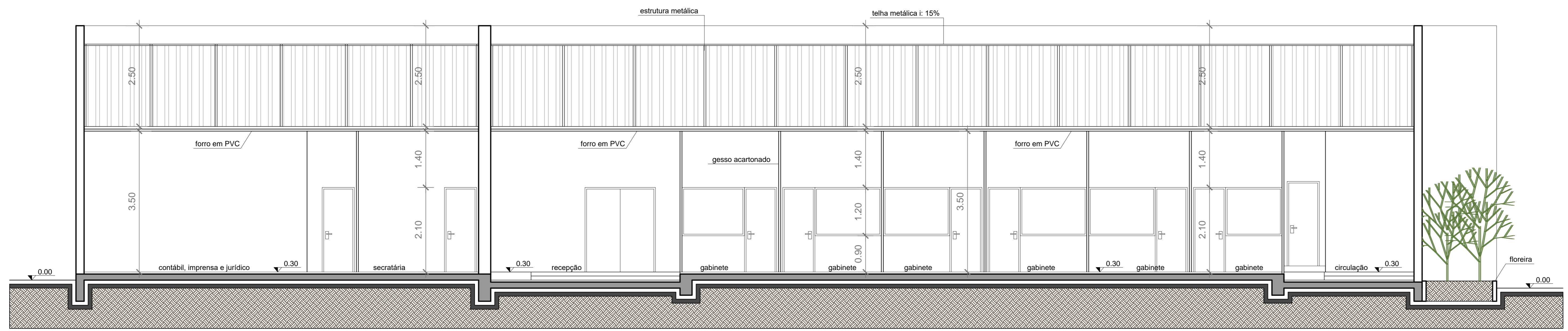
Corte BB' esc: 1/50
